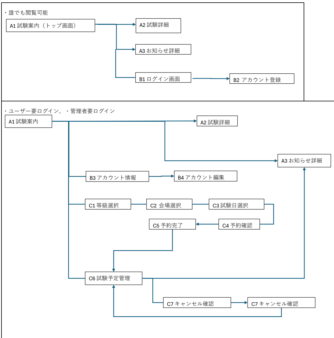
画面遷移図
